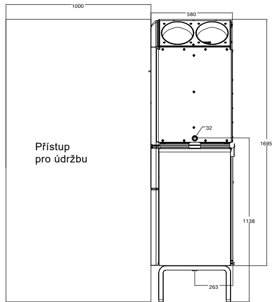
Boční pohled
