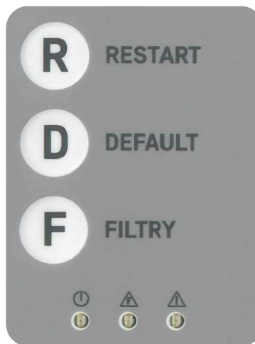
Obrázek 2: Ovládací panel zařízení „Ventbox“
