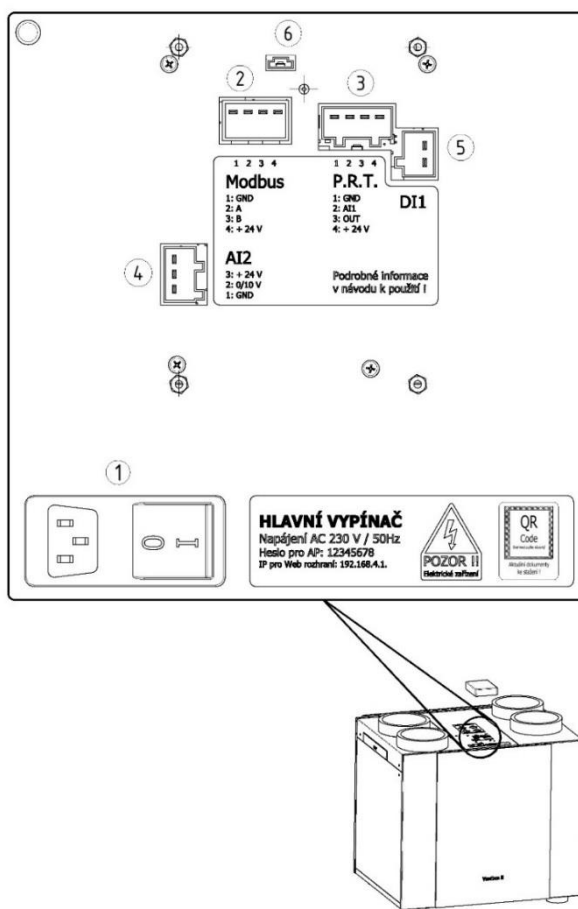
Obrázek 34: Panel řízení s připojením pro konektory
