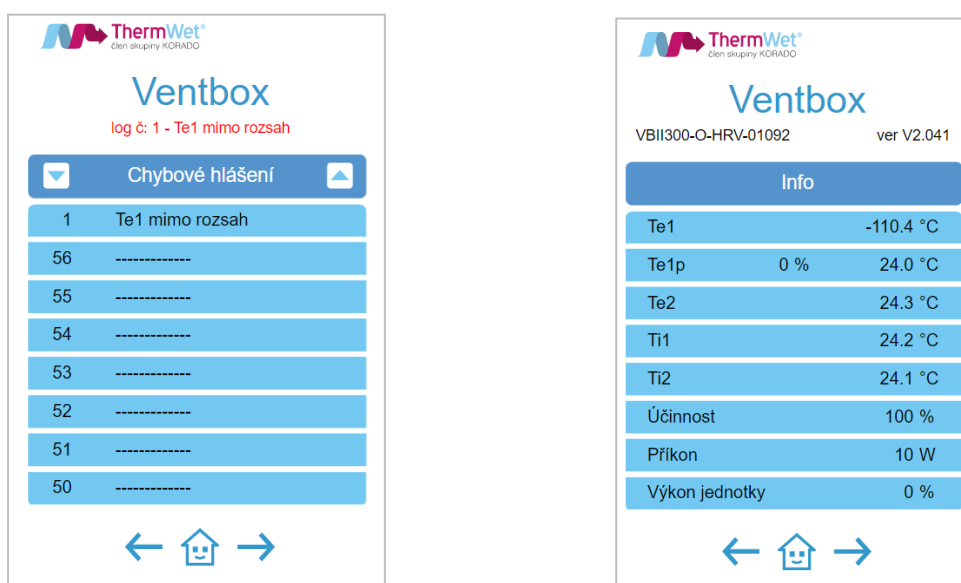
Obrázek 30: Indikace poruchy – Chybové hlášení / Info panel-teplota čidla_Te1
