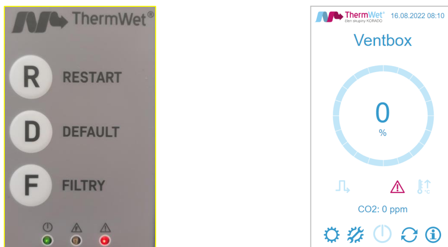
Obrázek 29: Indikace poruchy – ovládací panel / úvodní obrazovka
